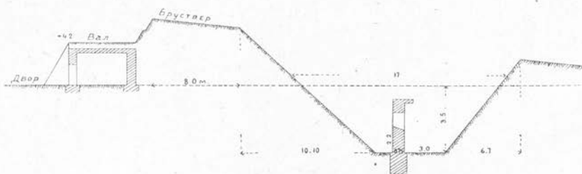
Профиль батареи.
