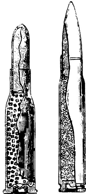
Старая тупая пуля.
