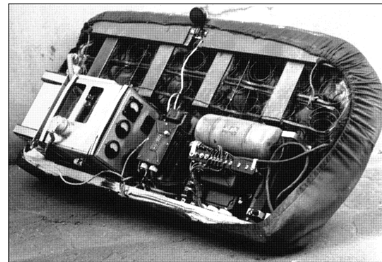
Радиостанция, замаскированная в автомобиле.
