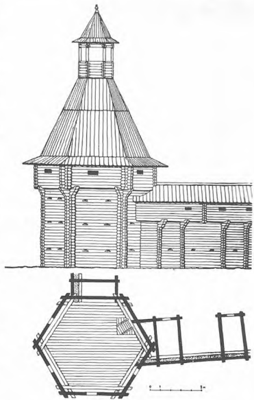
Угловая башня Олонецкой крепости. XVII в. План-реконструкция
