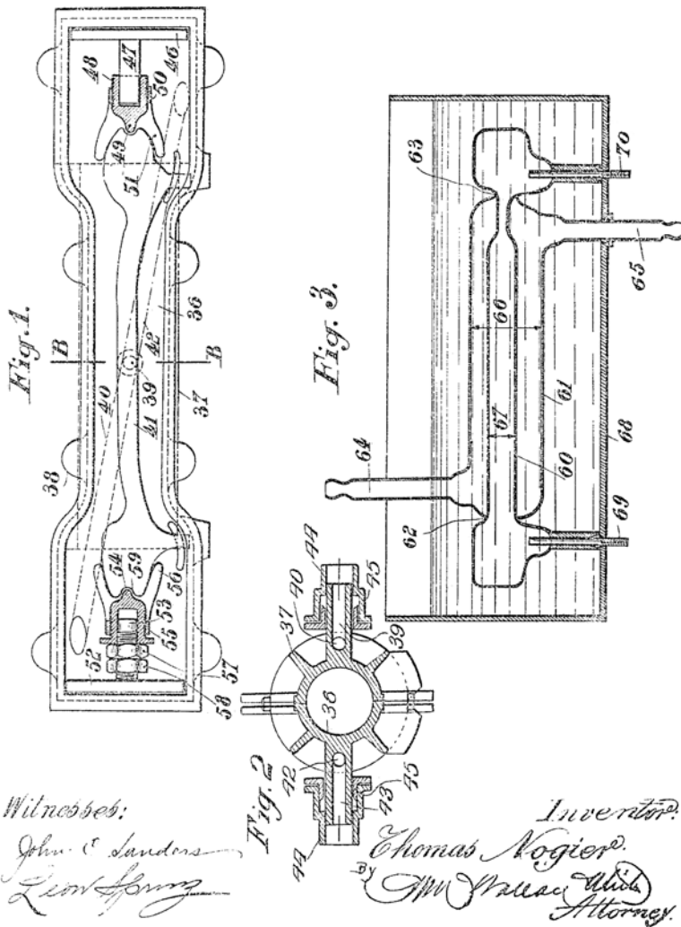
Схема устройства аппарата Ноже для стерилизации воды, прилагавшаяся к патенту на изобретение
