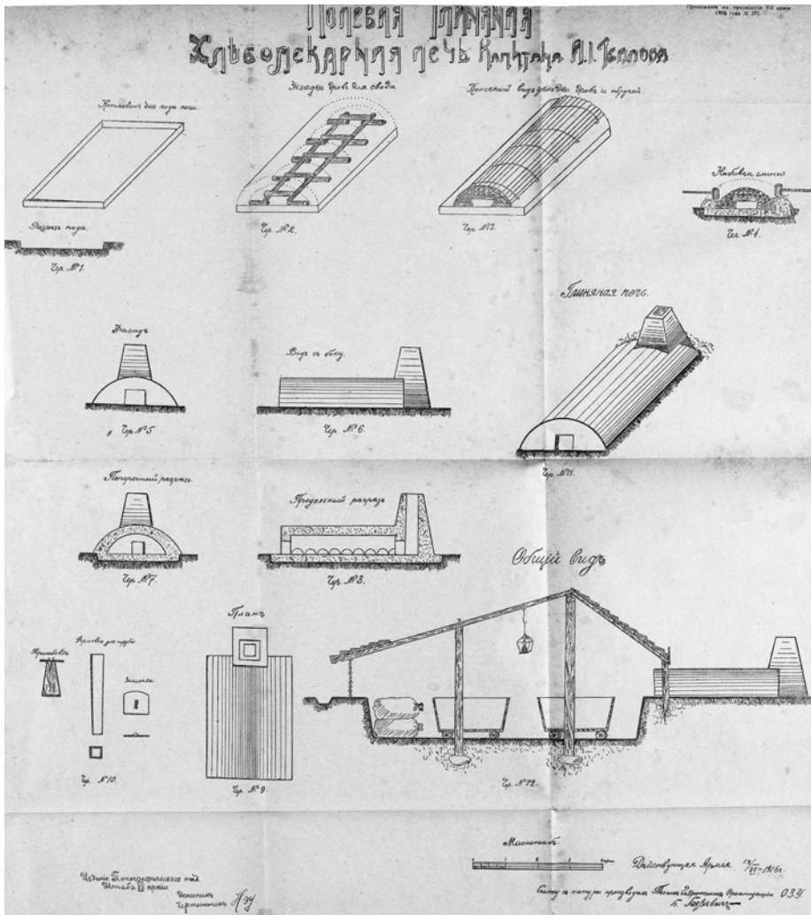
Эскиз полевой глиняной хлебобулочной печи капитана А. И. Теплова. Ее конструкция была столь удачной, что использовалась бойцами Красной армии в ходе советско-польской войны 1919–1921 годов
