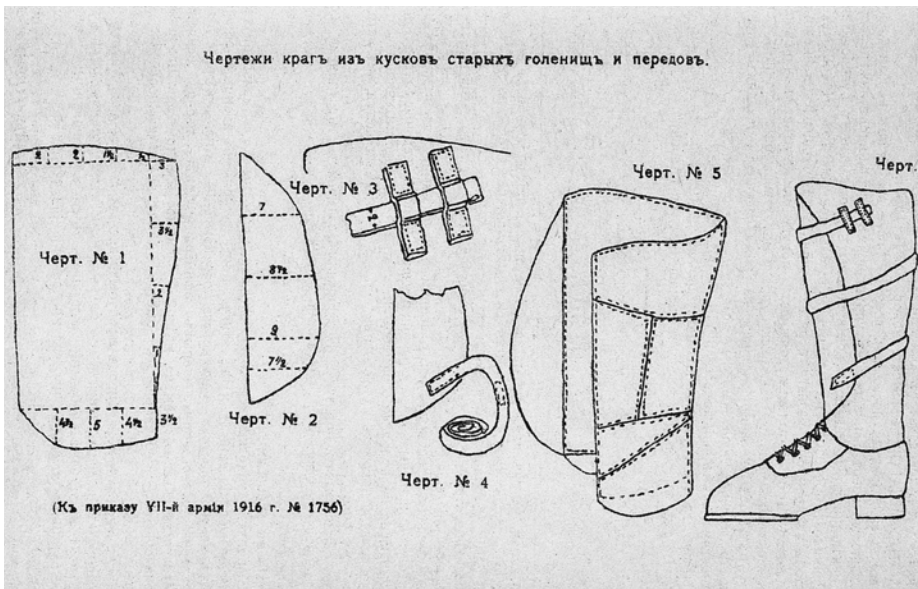
Чертежи краг из кусков старых голенищ и передов
