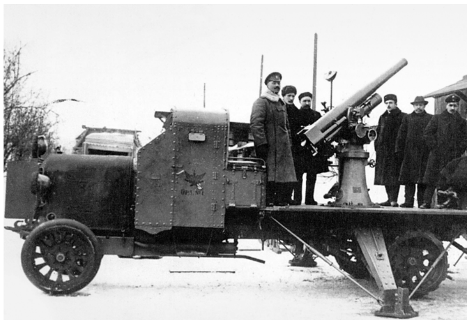
Первое русское противоаэропланное 76-мм орудие образца 1914 года, пушка Тарновского-Лендера на шасси броневедомокола «Руссо-Балт» тип Т. Крайний слева на фото — штабс-капитан В. В. Тарновский
