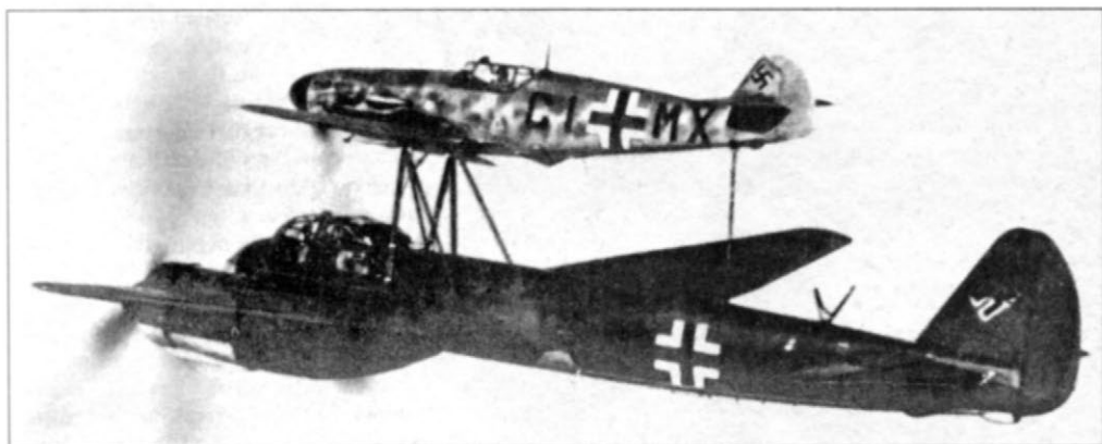
Испытания самолета-снаряда «Мистель» S1 в 1943 году. В качестве носителя боезаряда использовался бомбардировщик Ju-88 А-4. Самолет управления — Me-109 F-4.
