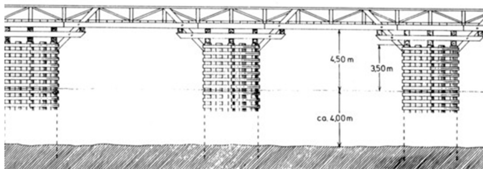
Реконструкция секции моста в Конфлуэнтесе
