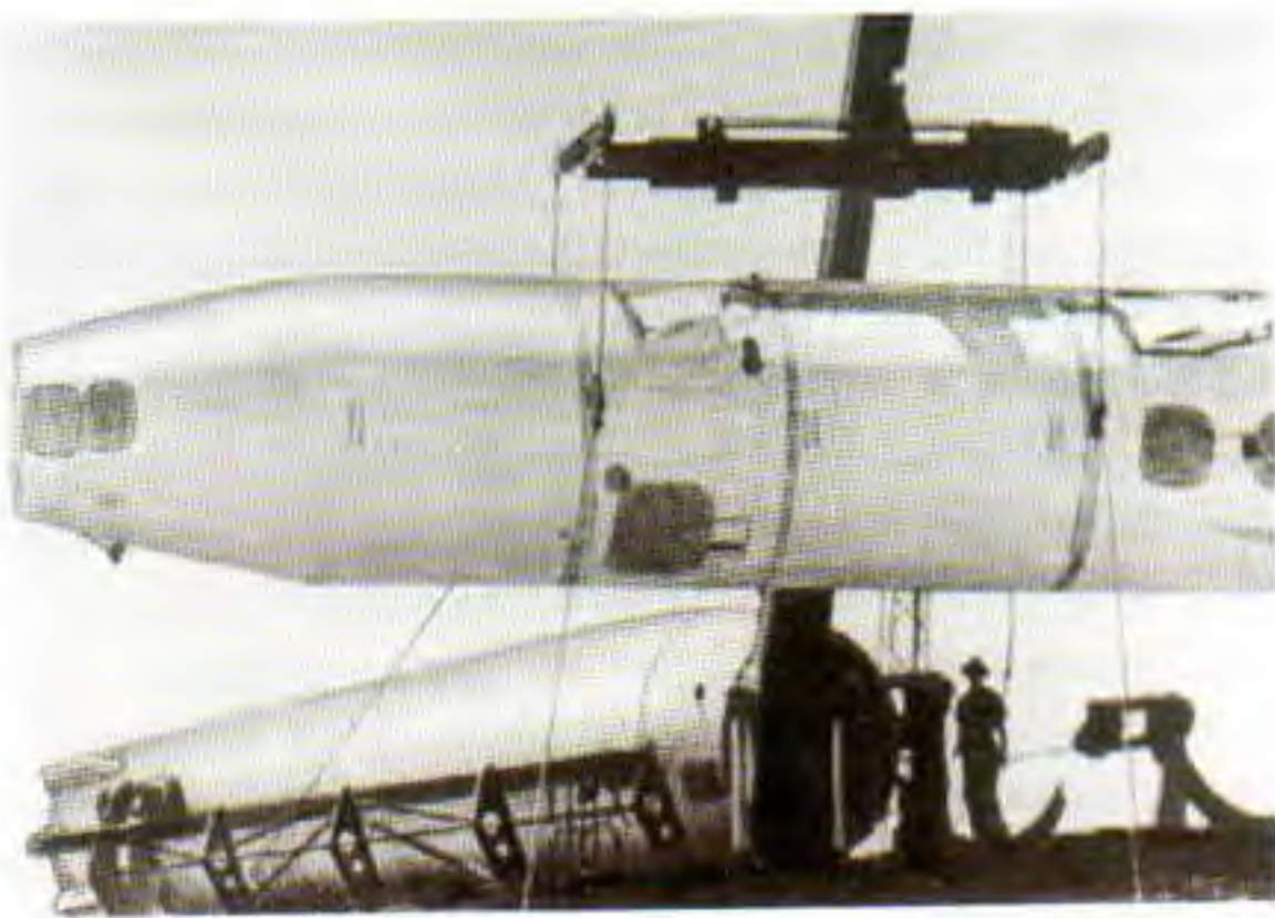
Ракета Р-16 (Р-16У) наземного базирования. Сборка ракеты
