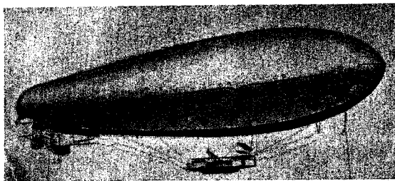
Морской дирижабль сист. Кронко (Италия. 1914). Объемъ 12.000 куб. м., скорость 70 килом., длина 83 м., поперечникъ 17 м., моторы 500 лош. силъ.
