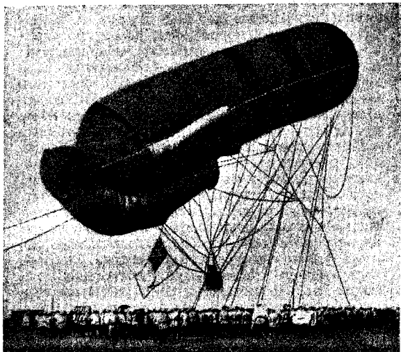
Змѣйковъй аэростатъ (Россія).
