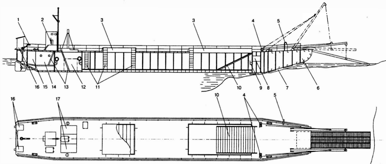
Самоходная десантная баржа-болиндер времен Первой мировой войны.
