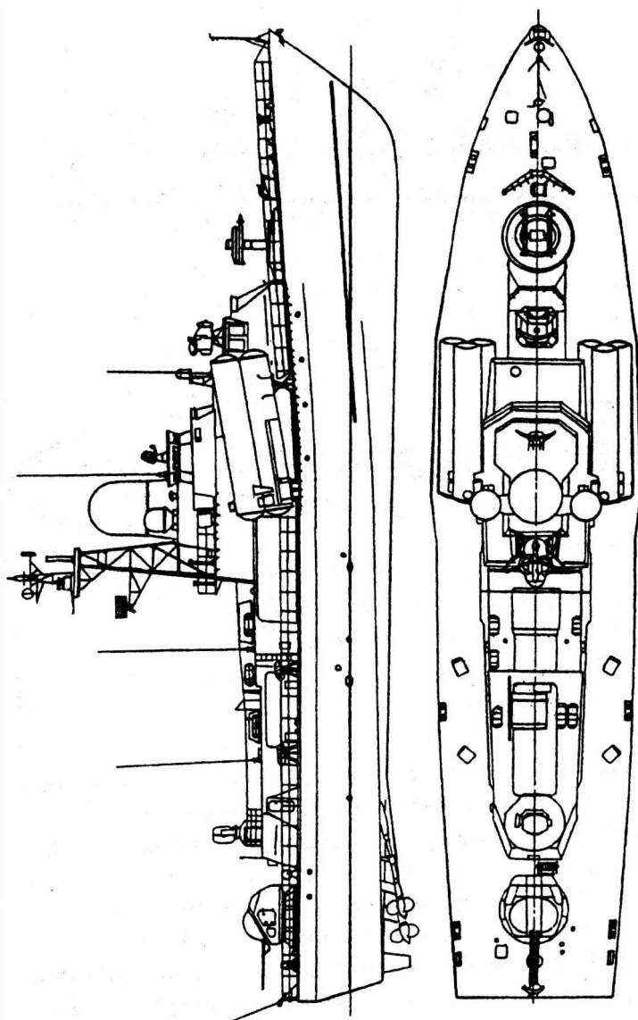
«Зарница» (проект 1234), 1970 г.
