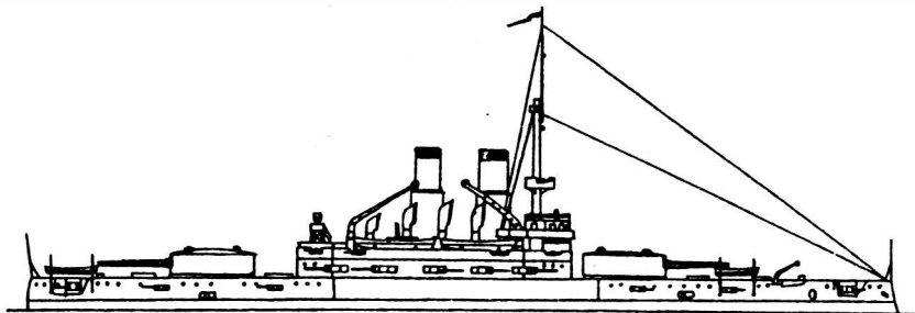
Так хотели переделать «Чесму», но деньги ушли на восстановление «Очакова»
