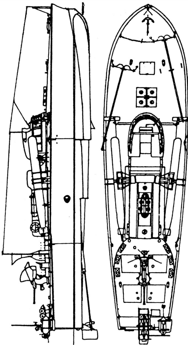
Итальянский торпедный катер «MAS»
