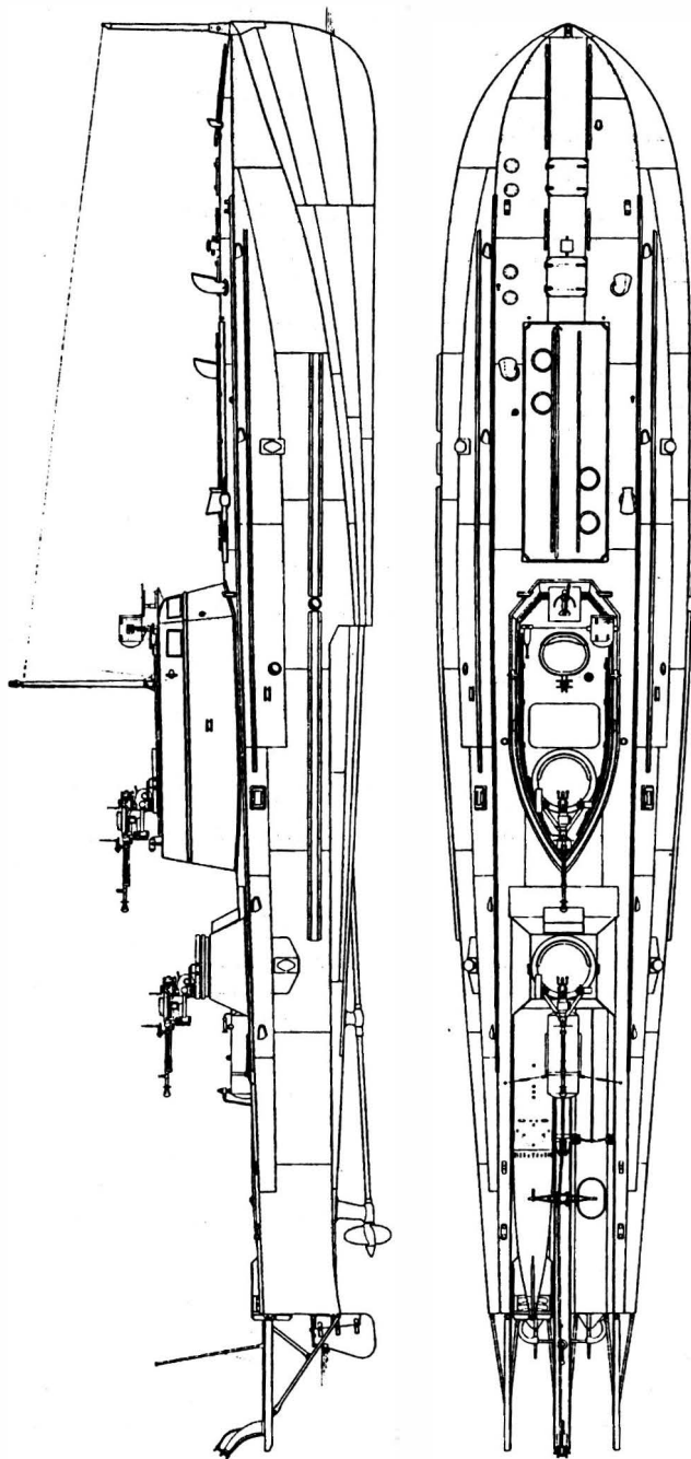
Советский торпедный катер типа Г-5
