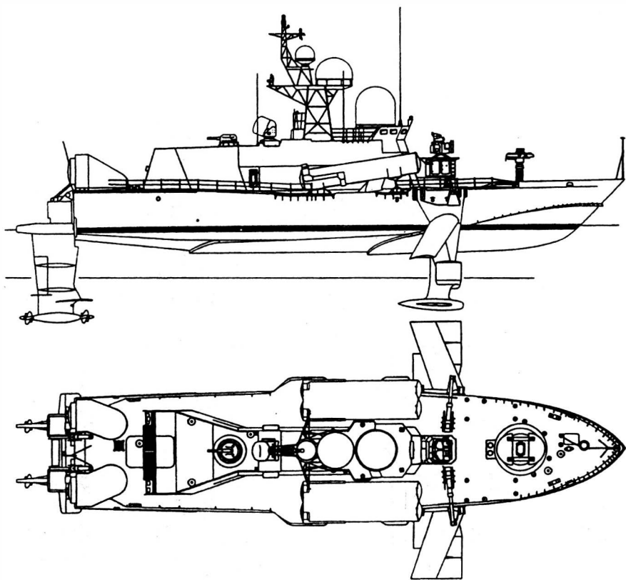
«МПК-5» (проект 1240), 1977 г.
