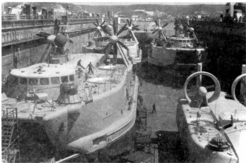
Суда на воздушной подушке в плавучем доке в Севастополе
