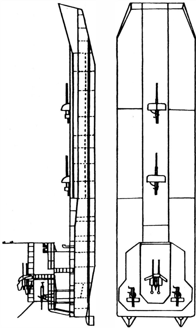
Германская артиллерийская баржа
