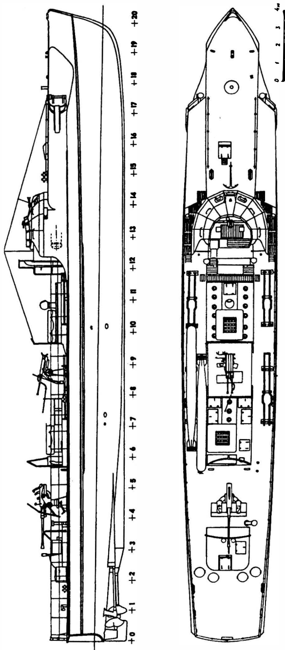
Германский торпедный катер «S-100»
