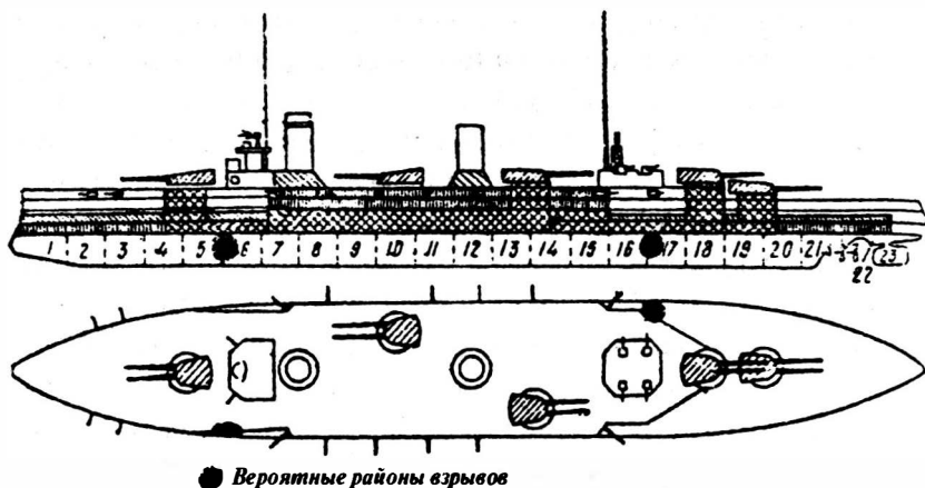
Схема повреждения линейного крейсера «Гебен» на русских минах у Босфора 26 декабря 1914 г.
