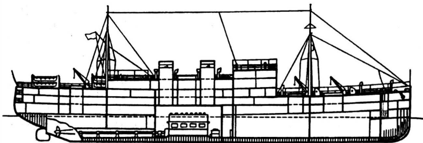
Теплоход «Армения». Продольный разрез.
