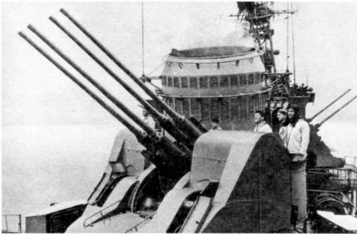
Зенитная установка на советском эсминце. 1970-е годы. Средиземное море. Зенитчики отслеживают пролет натовского самолета. Есть версия, что однажды в такой ситуации у матросика не выдержали нервы и он нажал на спусковую педаль. Загрохотала счетверенная установка, а патрульный «Нептун» развалился в воздухе. Инцидент замяли
