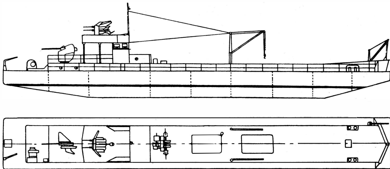
Германский быстроходный транспорт типа «F» (после войны использовались в советском флоте под названием «большие десантные баржи»).
