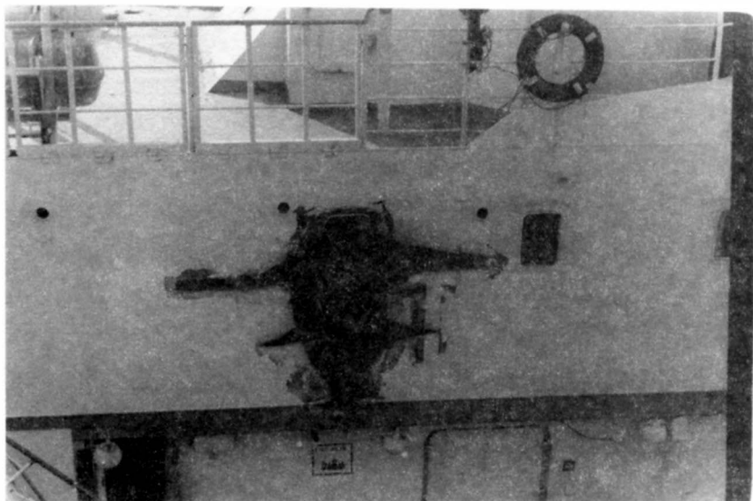
Входное отверстие от ракеты П-35 в борту парохода «Верещагино». Ракета имела инертную боевую часть
