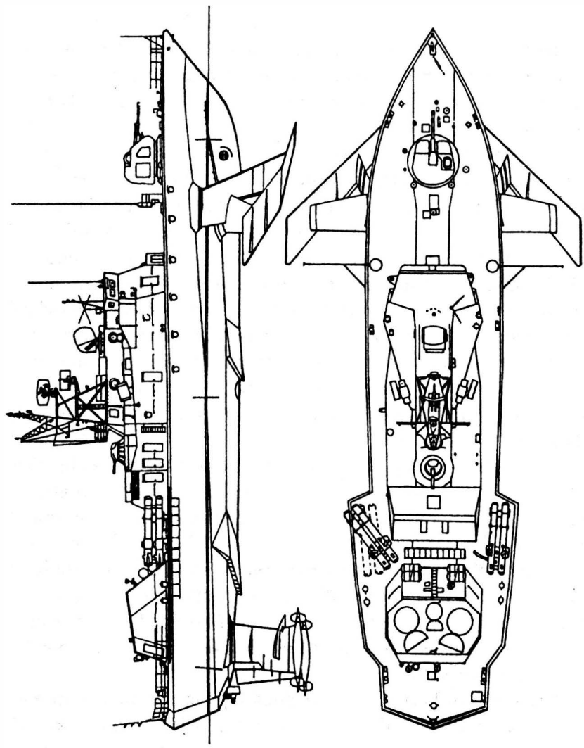
Малый противолодочный корабль «МПК-215» (проект 11451), 1987 г.
