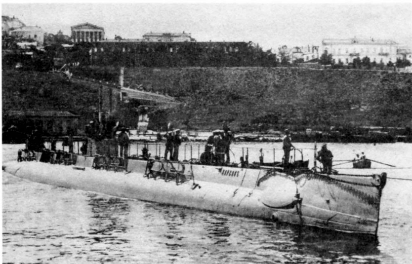
Подводная лодка «Нарвал» в Севастополе
