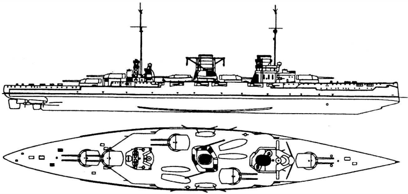
Линейный крейсер «Гeben»
