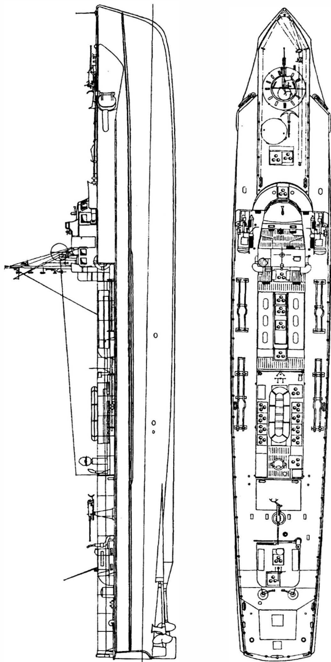
Торпедный катер «S-100» с бронированной рубкой
