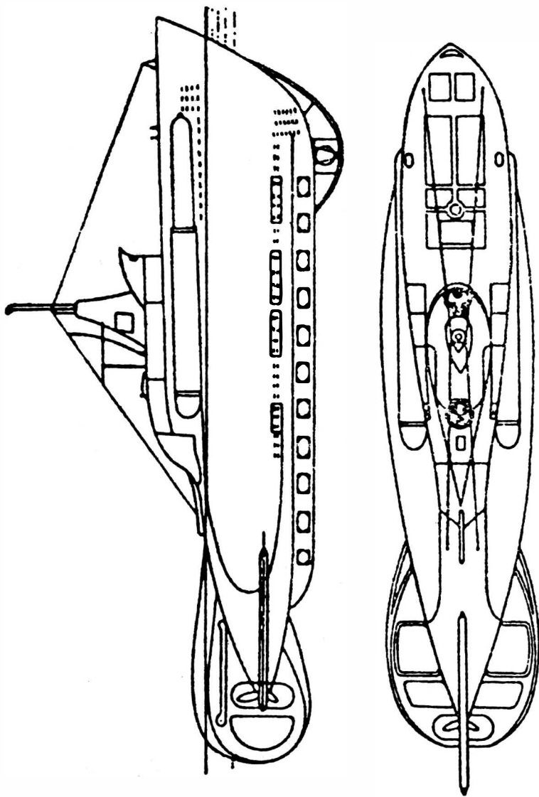
Итальянская сверхмалая подводная лодка типа «СВ»
