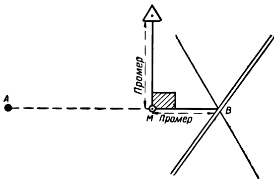
Рис. 39. Привязка наблюдательного пункта по перпендикуляру к створу с двумя промерами
