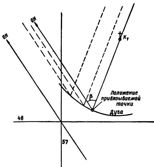
Рис. 46. Привязка наблюдательного пункта при помощи дальномера, ориентированного в основном направлении
