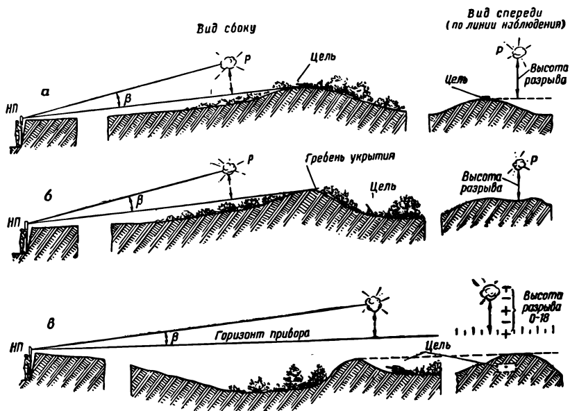
Рис. 89. Измерение высоты разрыба:
