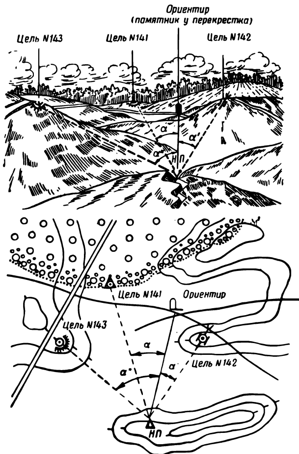
Рис. 81. Определение положения цели на карте, когда цель расположена на резко выраженном рубеже: вверху — вид местности с наблюдательного пункта; внизу — нанесение на карту целей, обнаруженных на этой местности
