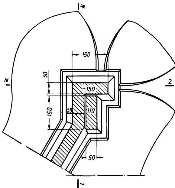
Рис. 70. Открытый вспомогательный наблюдательный пункт (передовой или боковой); время на отрывку 10 человеко-часов
