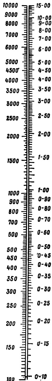
Рис. 113 Номограмма для определения дальности до цели
