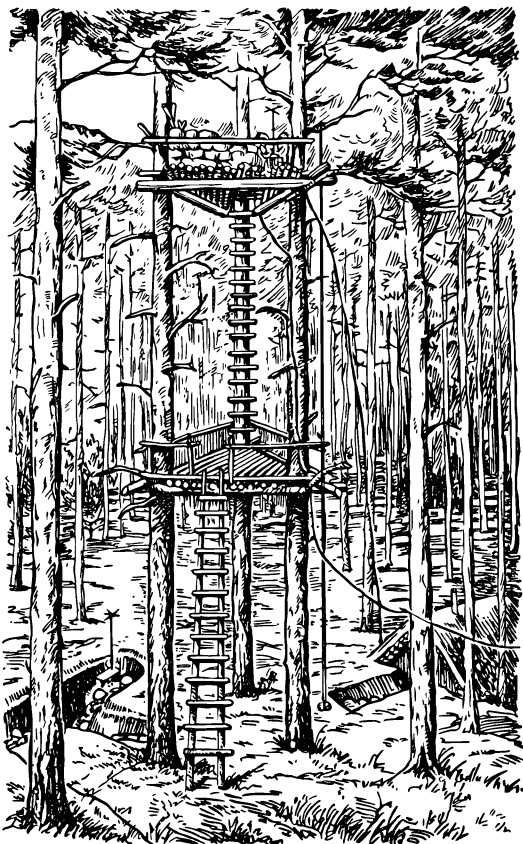
Рис. 62. Основной наблюдательный пункт на вышке, укрепленной на трех деревьях
