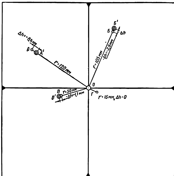
Рис. 59. К примерам введения поправок за рельеф: A, B, B, \Gamma — положение точек на аэроснимке; A', B', B' — исправленное положение тех же точек на снимке после введения поправок за рельеф; в положение точки \Gamma поправка не вводится
