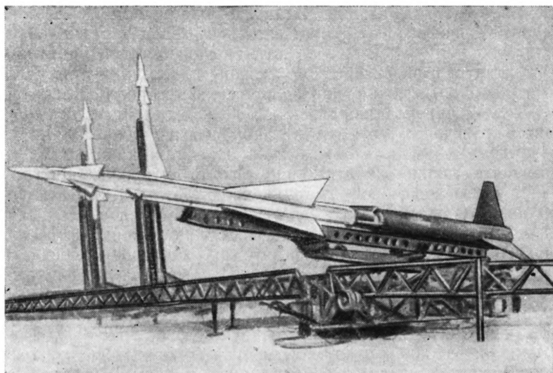
Рис. 25. Зенитный управляемый реактивный снаряд (зенитная ракета) «Найк», подготавливаемый к пуску; на заднем плане — другой такой же снаряд, подготовленный к пуску (диаметр 1,5 м, стартовый вес 450 кг, дальность полета 27 км, досягаемость по высоте 23 км, а в варианте «Найк-Геркулес» соответственно 120 км и около 30 км)
