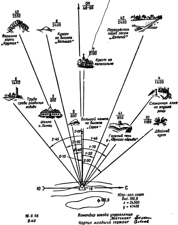
Рис. 85. Пример схемы ориентиров батареи:
