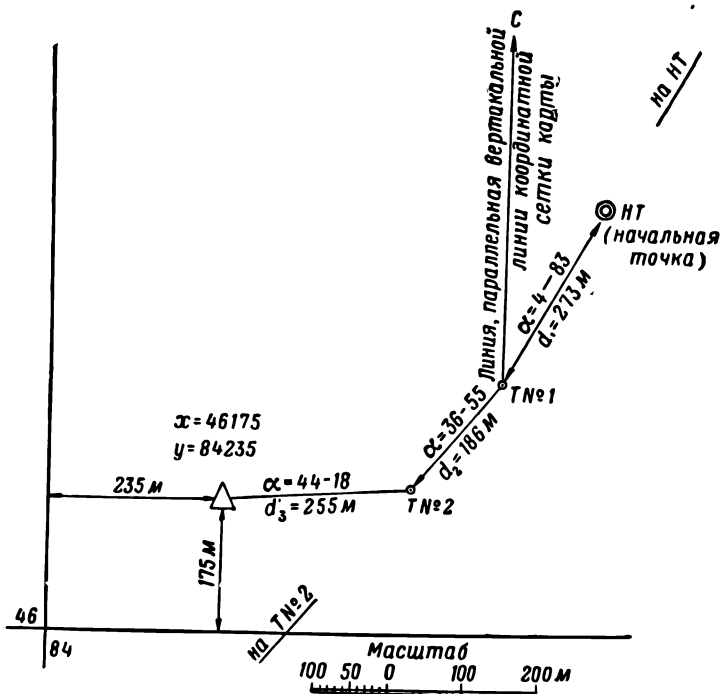
Рис. 44. Пример привязки наблюдательного пункта ходом
