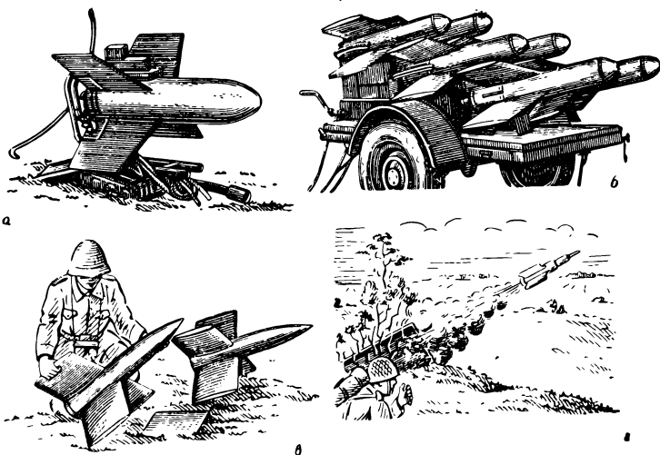
Рис. 5. Противотанковые управляемые реактивные снаряды: а — «SS-10»; б — «SS-11» на колесной пусковой установке на 6 снарядов; в — установка снарядов «Москито» на огневой позиции; г — момент выстрела снарядом «Виккерс — Армстронг 891»
