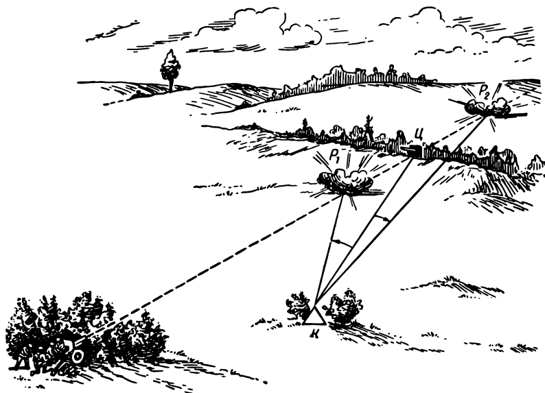
Рис. 97. Если наблюдательный пункт смещен в сторону от плоскости стрельбы, недолеты кажутся отклонениями в сторону огневой позиции, перелеты — отклонениями в противоположную сторону
