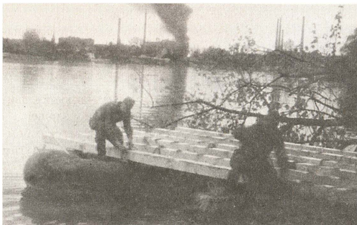
Наведение понтонного моста
