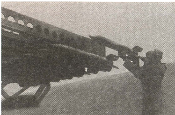
Установка реактивных снарядов на направляющие БМ-13
