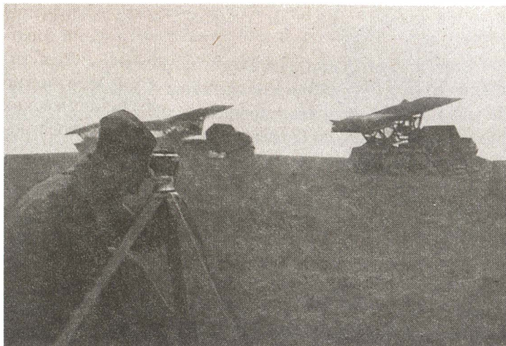
Топографическая привязка позиции и установка в основное направление БМ-13
