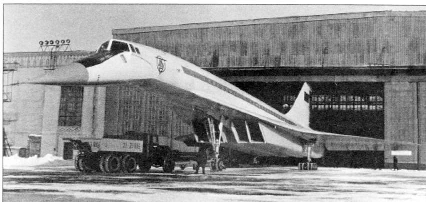
Выкатка из цеха опытного самолета Ту-144
