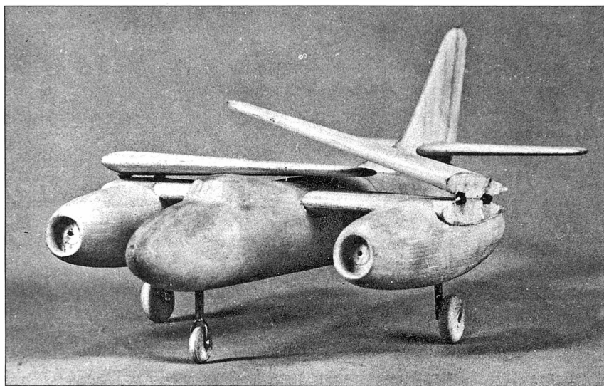
Модель самолета «509»
