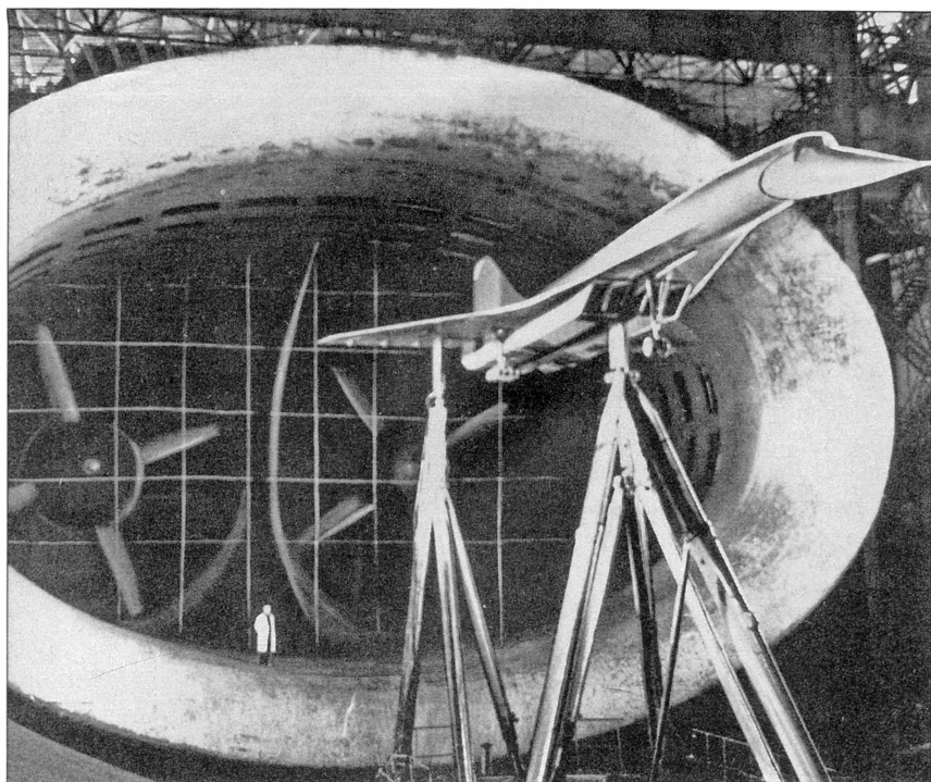
Продувка модели опытного самолета Ту-144 в аэродинамической трубе ЦАГИ
