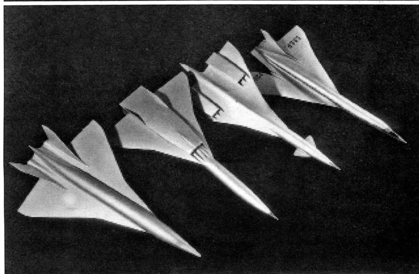
Модели различных вариантов компоновки СПС Ту-144
