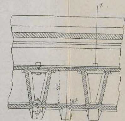
Горизонтальной чертёж горизонтальной апарей.
