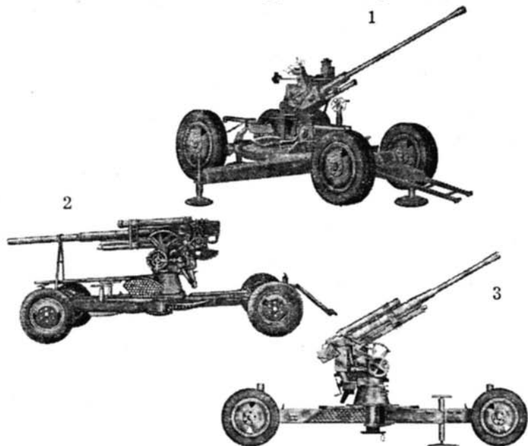
Рис. 7. Зенитные орудия: 1 — 37-мм автоматическая зенитная пушка; 2 — 76-мм зенитная пушка; 3 — 85-мм полуавтоматическая зенитная пушка.
