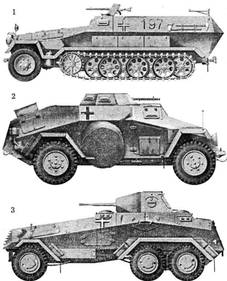
Рис. 11. Основные виды бронемашин и бронеевтомобилей войск вермахта на 22 июня 1941 года: 1 — средний бронетранспортер (специальная машина 251); 2 — легкий разведывательный бронеевтомобиль (специальная машина 222); 3 — тяжелый трехосный бронеевтомобиль (специальная машина 231/232).
