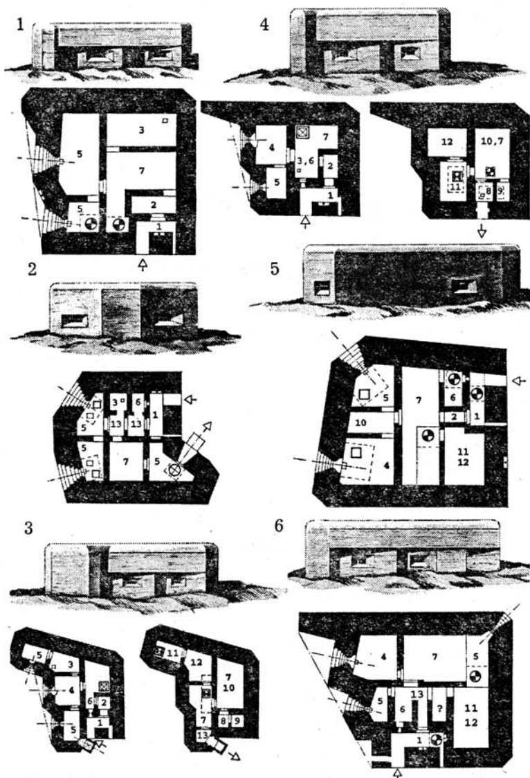
Рис. 8. Основные долговременные сооружения укрепрайонов западной границы СССР:
