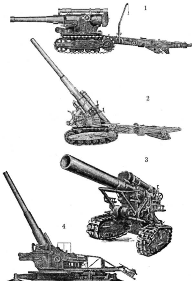
Рис. 4. Основные марки артиллерийских орудий большой мощности, состоявших на вооружении в артиллерийских частях ПриОВО: 1 — 203-мм гаубица (Б-4) большой мощности; 2 — 152-мм пушка Бр-2; 3 — 280-мм орудие Бр-5; 4 — 210-мм дальнобойная пушка Бр-17.
