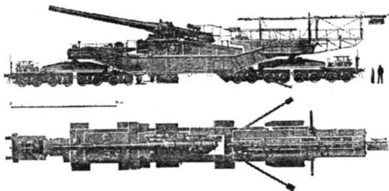
Рис. 5. 305-мм гаубица, установленная на транспортере ТМ-2-12.
