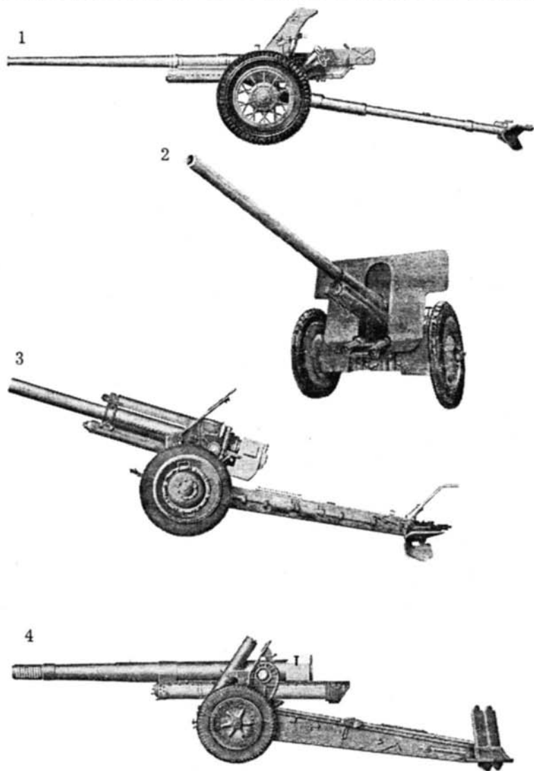
Рис. 3. Основные марки артиллерийских систем, имевшихся на вооружении в артиллерийских частях ПриБОВО: 1 — 45-мм противотанковая пушка; 2 — 76-мм дивизионная пушка; 3 — 122-мм гаубица; 4 — 152-мм гаубица-пушка;
