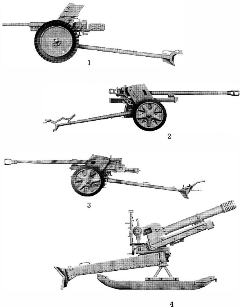
Рис. 12. Основные образцы артиллерийских систем вермахта на 22 июня 1941 г.:
