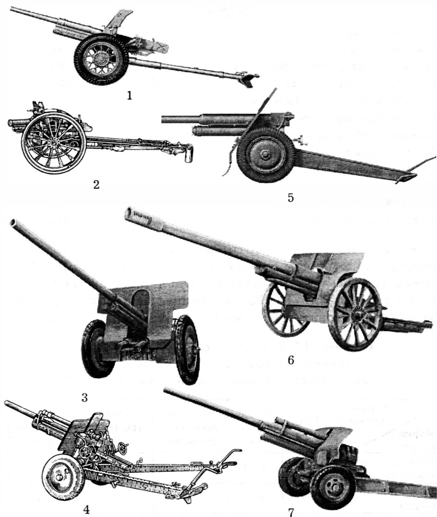
Рис. 5. Артиллерийские системы, находившиеся на вооружении войск КОВО на 22 июня 1941 г.:
