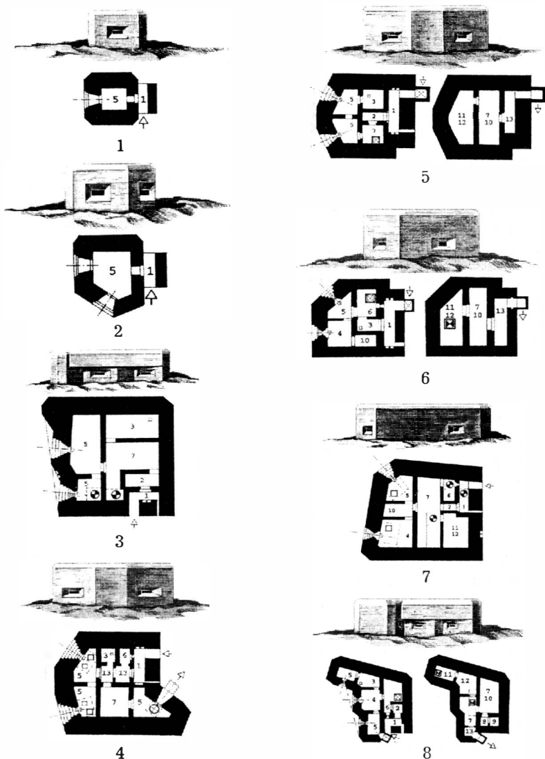
Рис. 8. Основные фортификационные сооружения западных укрепрайонов СССР:
