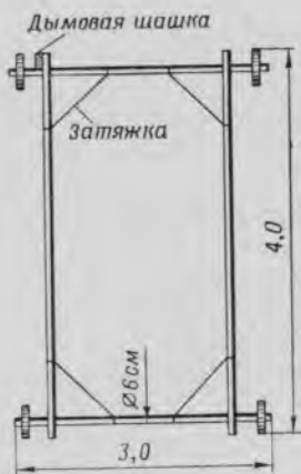
Подвижная рама из жердей на деревянных роликах
