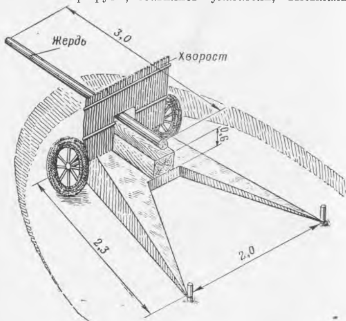
Макет 76-мм орудия
