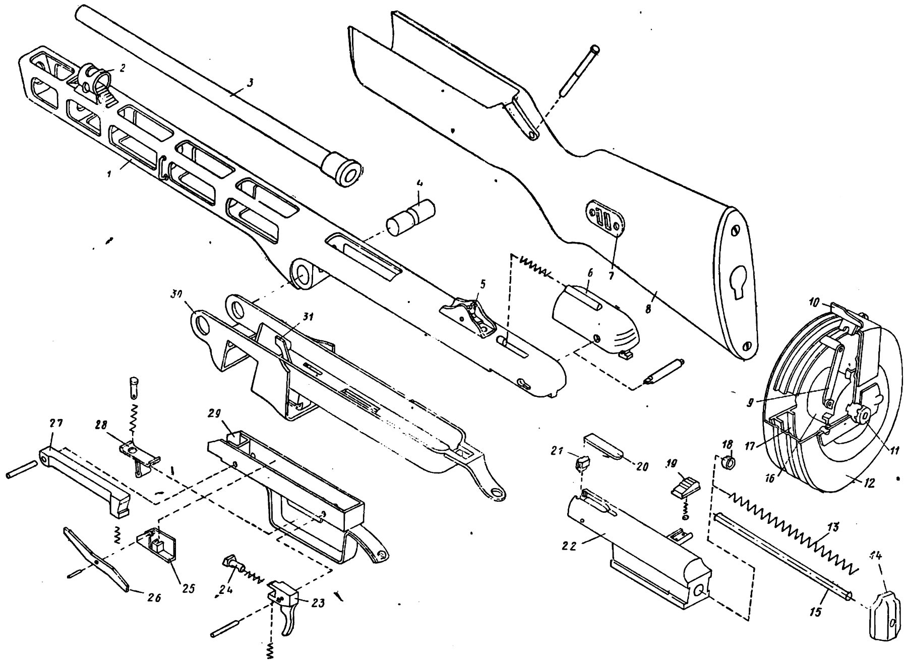
Рис. 111.2. Детали и сборки пистолета-пулемета Шпагина:
