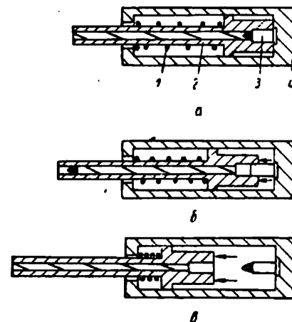
Рис. 1.25. Схема автоматического оружия, работающего на принципе использования силы врезания пули в нарезы: 1 — возвратная пружина; 2 — ствол; 3 — патрон; 4 — затвор (затворная коробка); а — положение в момент разбития капсюля; б — движение пули по каналу ствола; в — накат ствола
