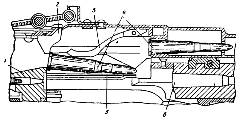
Рис. I.12. Конструктивная схема обратной подачи патрона: 1 — досылатель затвора; 2 — копир; 3 — подаватель патрона; 4 — патрон; 5 — приемное окно; 6 — патронник
