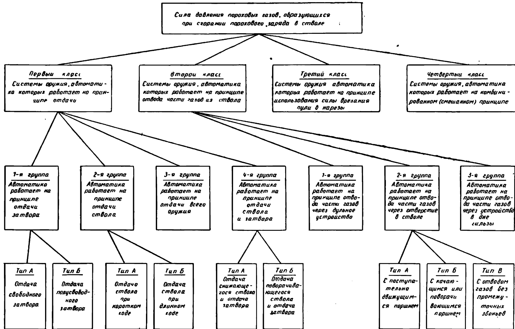
Рис. 1.18. Классификация автоматического оружия по принципу работы автоматики
