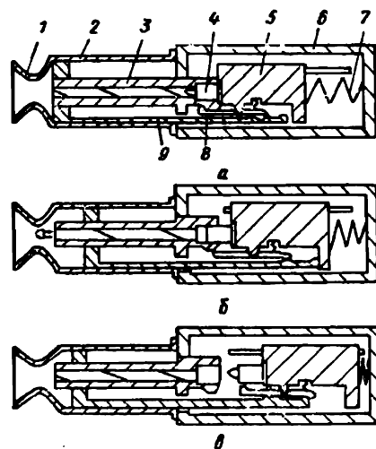
Рис. 1.23. Схема автоматического оружия, работающего на принципе отвода части пороховых газов через дульное устройство: 1 — дульное устройство; 2 — кожух ствола; 3 — ствол; 4 — патрон; 5 — затвор; 6 — ствольная коробка; 7 — возвратная пружина; 8 — запирающий рычаг; 9 — затворная рама с штыком и поршнем
