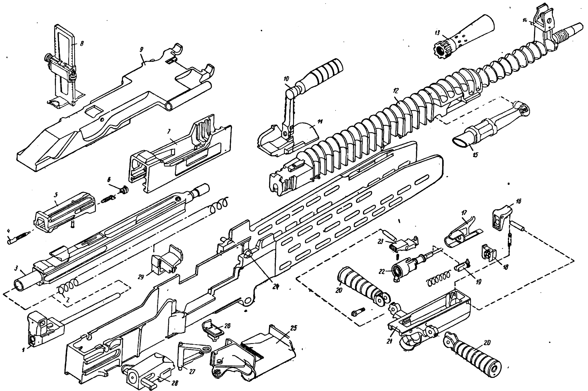
Рис. VI.6. Детали и сборки пулемета ZB53:
