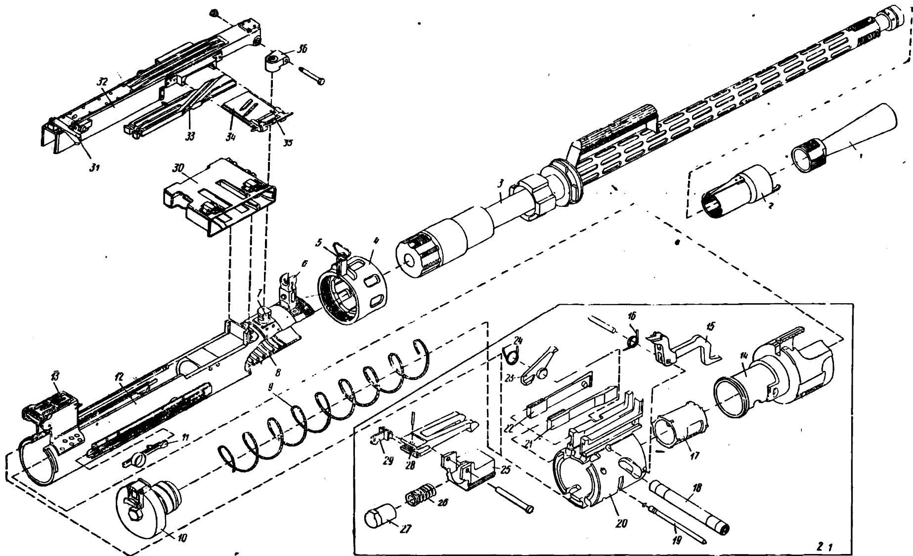
Рис. VII.4. Детали и сборки пулемета КПВ:
