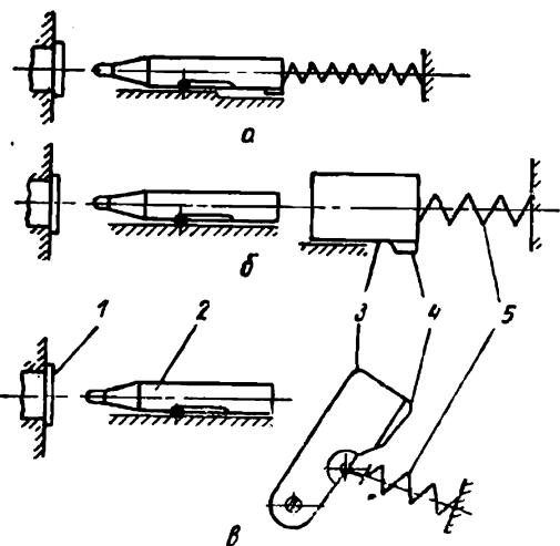
Рис. 1.4. Схема ударникового (а) и курковых ударных механизмов с поступательным (б) и вращающимся (в) курками: 1 — гильза с капсюлем-воспламенителем; 2 — ударник; 3 — курок; 4 — боевой взвод; 5 — боевая пружина
