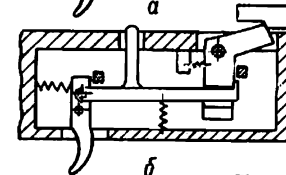
Рис. 1.5. Схемы спусковых механизмов:
