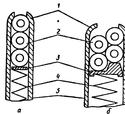
Рис. 1.6. Конструктивные схемы коробчатых магазинов с однорядным (а) и двухрядным (б) расположением патронов: 1 — загибы; 2 — патроны; 3 — подаватели патронов; 4 — подающие пружины; 5 — корпуса магазинов
