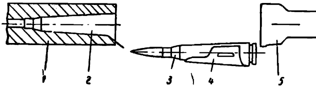
Рис. I.11. Схема прямого досылания патрона из ленты: 1 — ствол; 2 — патронник; 3 — патрон; 4 — незамкнутое звено ленты; 5 — досылатель затвора
