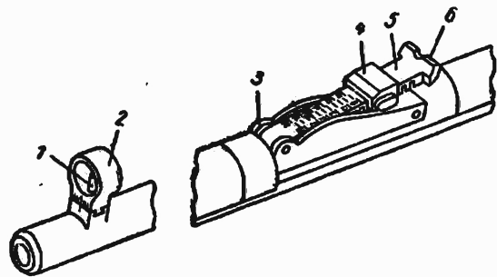
Рис. 1.14. Механическое прицельное приспособление: 1 — мушка; 2 — предохранитель мушки; 3 — основание прицела; 4 — хомут; 5 — прицельная планка; 6 — визир
