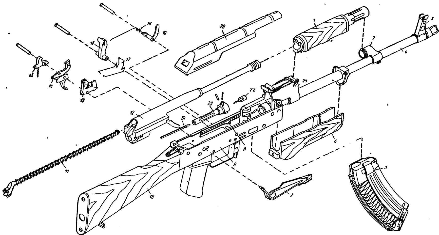
Рис. IV.2. Детали и сборки автомата АКМ:
