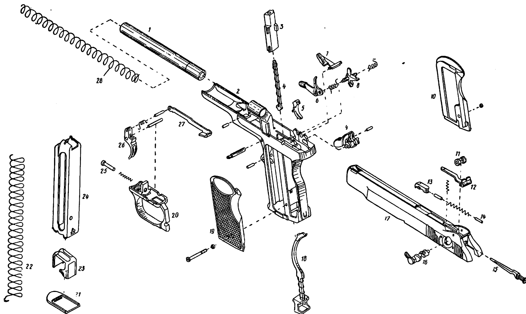
Рис. 11.5. Детали и сборки пистолета Стечкина:
