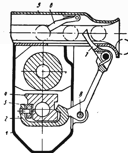
Рис. 1.9. Конструктивная схема механизма подачи ленты качающимся рычагом: 1 — ствольная коробка; 2 — рычаг подачи; 3, 8 — ролик и ось рычага; 4 — затворная рама с кулачковым приводом; 5 — приемник; 6, 7 — фиксирующий и подающий пальцы
