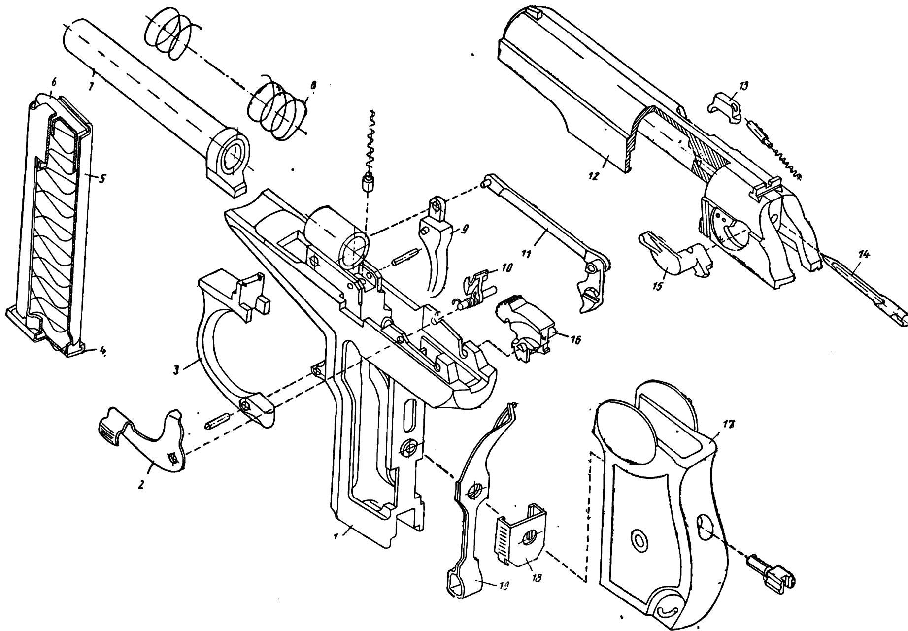
Рис. 11.2. Детали и сборки пистолета Макарова:
