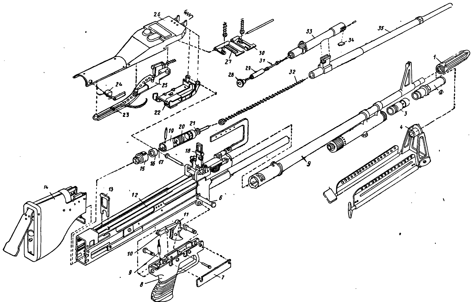
Рис. VI.18. Детали и сборки пулемета М60:
