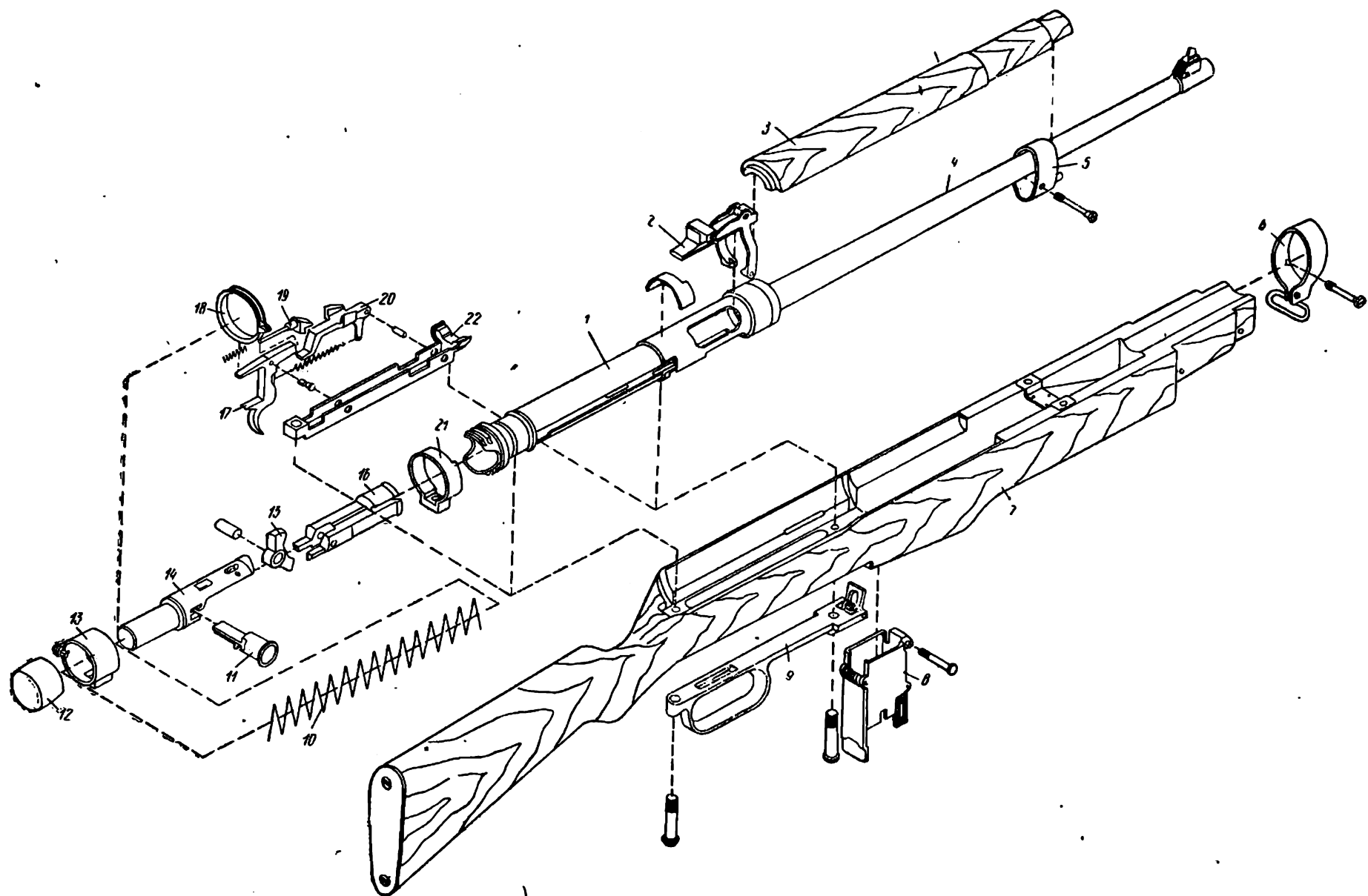
Рис. IV.11. Детали и сборки автоматического карабина 39М:
