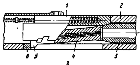
Рис. 1.3. Конструктивные схемы неподвижного (а), поперечно-движущегося клинового (б), качающегося (в) и продольно-скользящего, запирающегося перекосом (г) затворов: 1 — затворная рама; 2 — ствольная коробка; 3 — ствол; 4 — затвор; 5 — боевой упор затвора; 6 — сменный упор ствольной коробки
