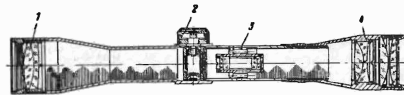
Рис. 1.15. Оптический прицел: 1 — объектив; 2 — механизм перемещения перекрестия; 3 — оборачивающая система линз; 4 — окуляр
