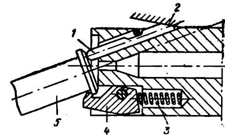
Рис. I.13. Схема удаления гильзы: 1 — подвижный жесткий отражатель; 2 — ствольная коробка; 3 — пружина выбрасывателя; 4 — выбрасыватель; 5 — гильза
