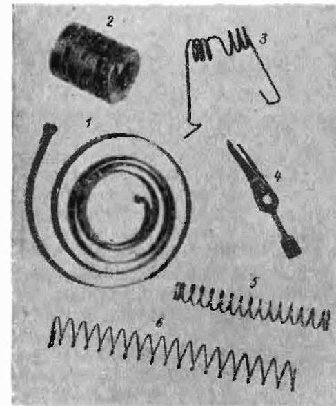
Рис. 1.17. Типы пружин: 1 — спиральная; 2 — буферная с прямоугольным сечением витков; 3 — кручения многожильная; 4 — пластинчатая; 5 — винтовая, цилиндрическая с круглым сечением; 6 — призматическая (коробчатых магазинов)
