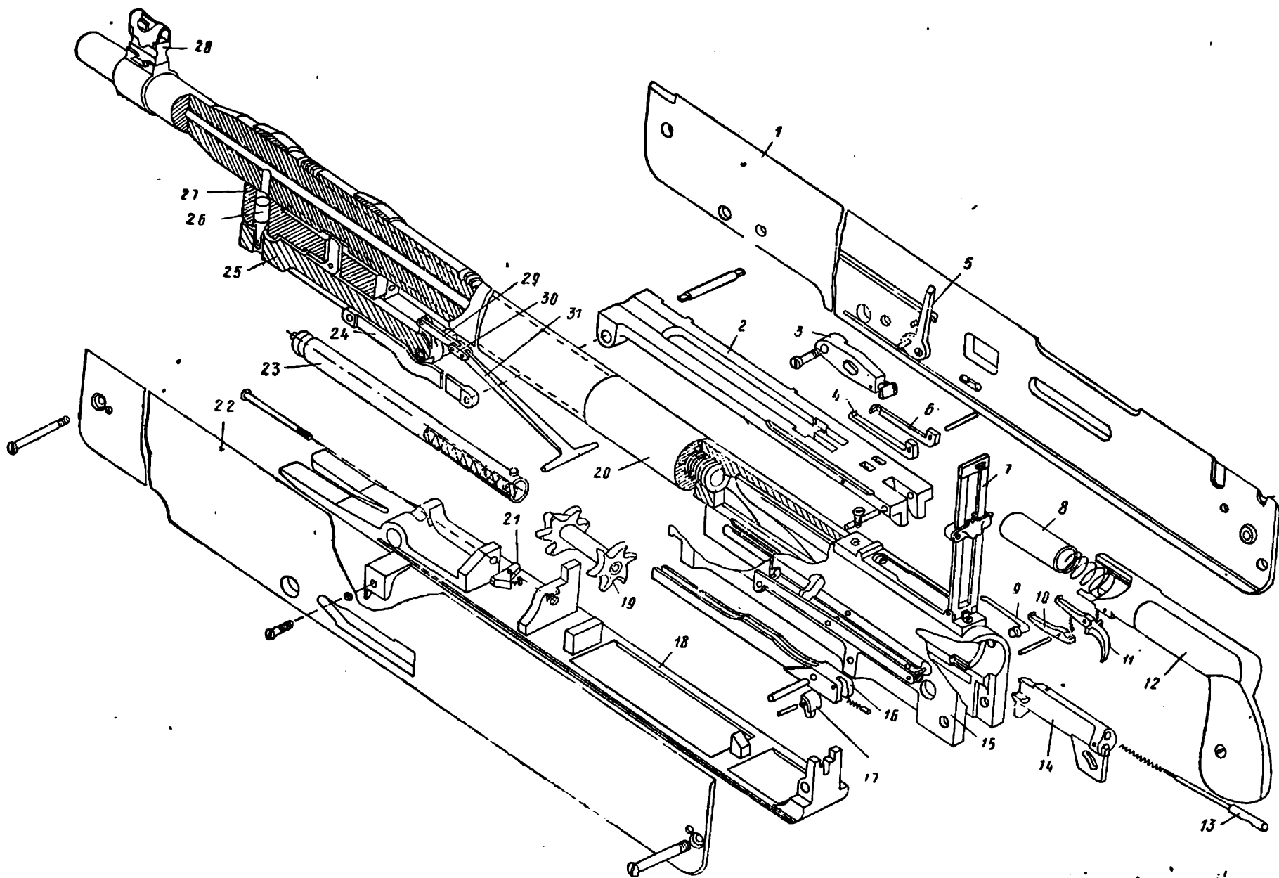
Рис. VI.8. Детали и сборки пулемета Колта:
