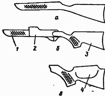
Рис. 1.16. Типы ложек: а — единая винтовочная с прямой шейкой; б — раздельная с пистолетной шейкой; в — приклад типа Монте-Карло с пистолетной шейкой; 1 — цевье; 2 — ствольная коробка; 3 — приклад; 4 — щека
