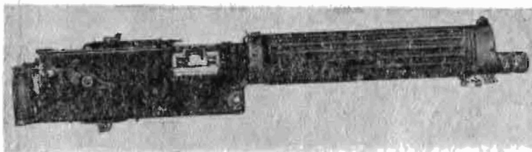
Рис. VI.1. Пулемет «Максим»
