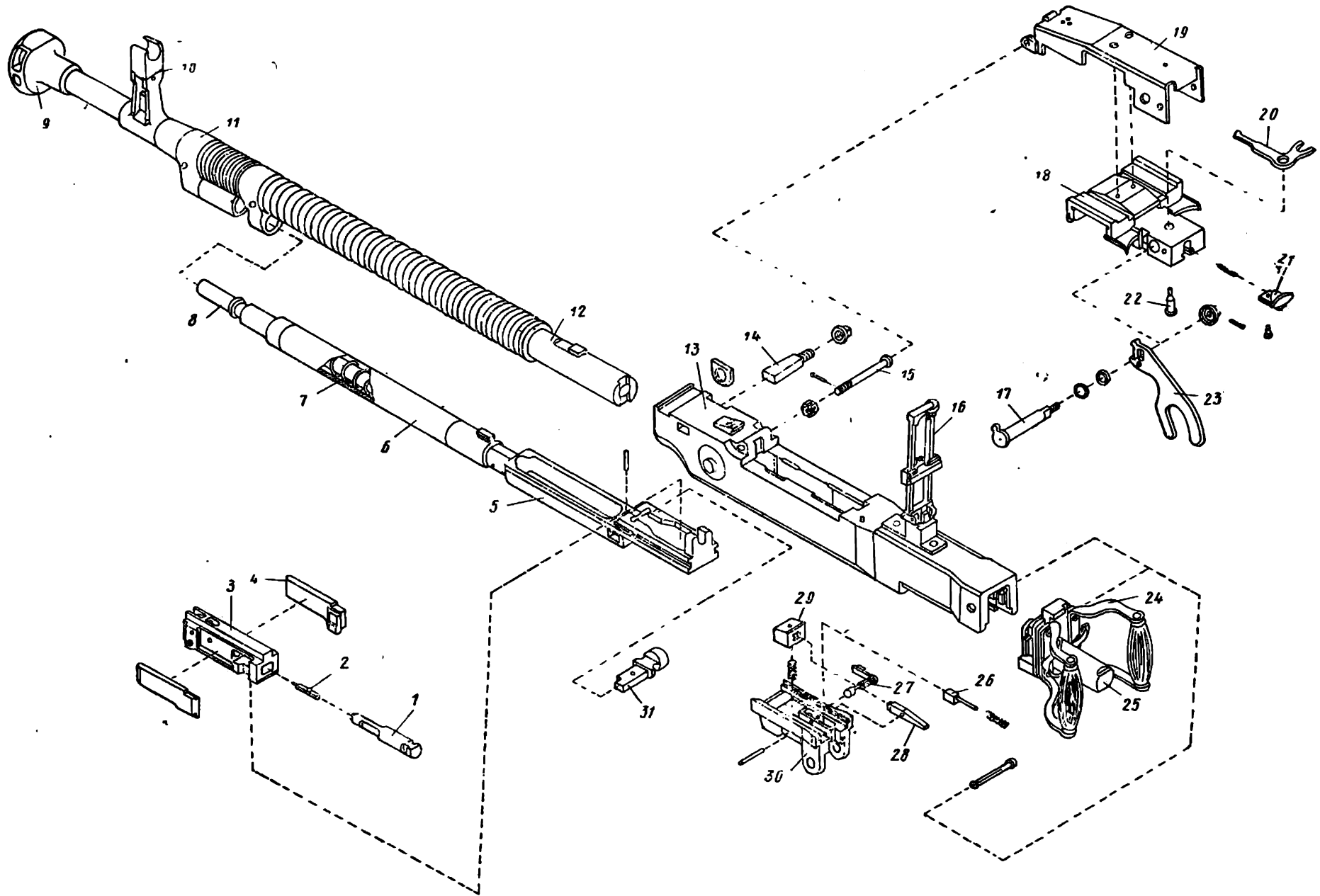
Рис. VII.2 Детали и сборки пулемета ДШКМ:
