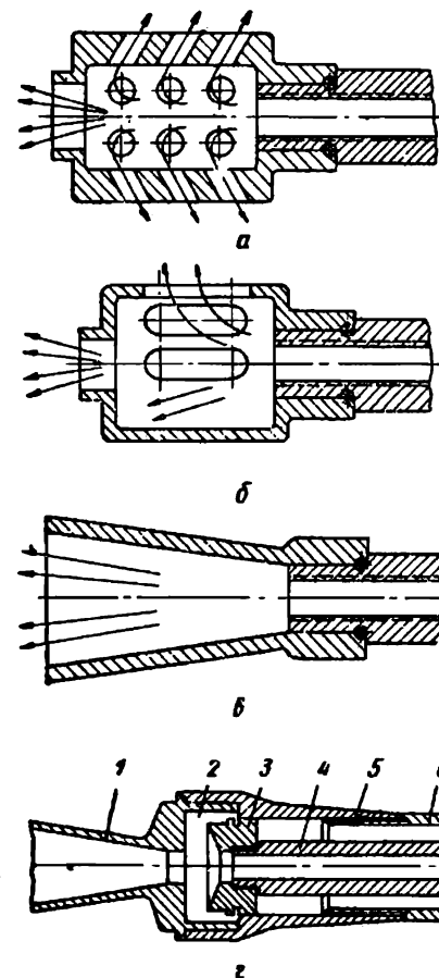
Рис. 1.2. Дульные устройства: а - дульный тормоз; б - тормоз-компенсатор; в - пламегаситель; г - усилитель отдачи с пламегасителем; 1 - муфта (пламегаситель); 2 - камера усилителя; 3 - поршень; 4 - ствол; 5 - корпус усилителя; 6 - кожух ствола
