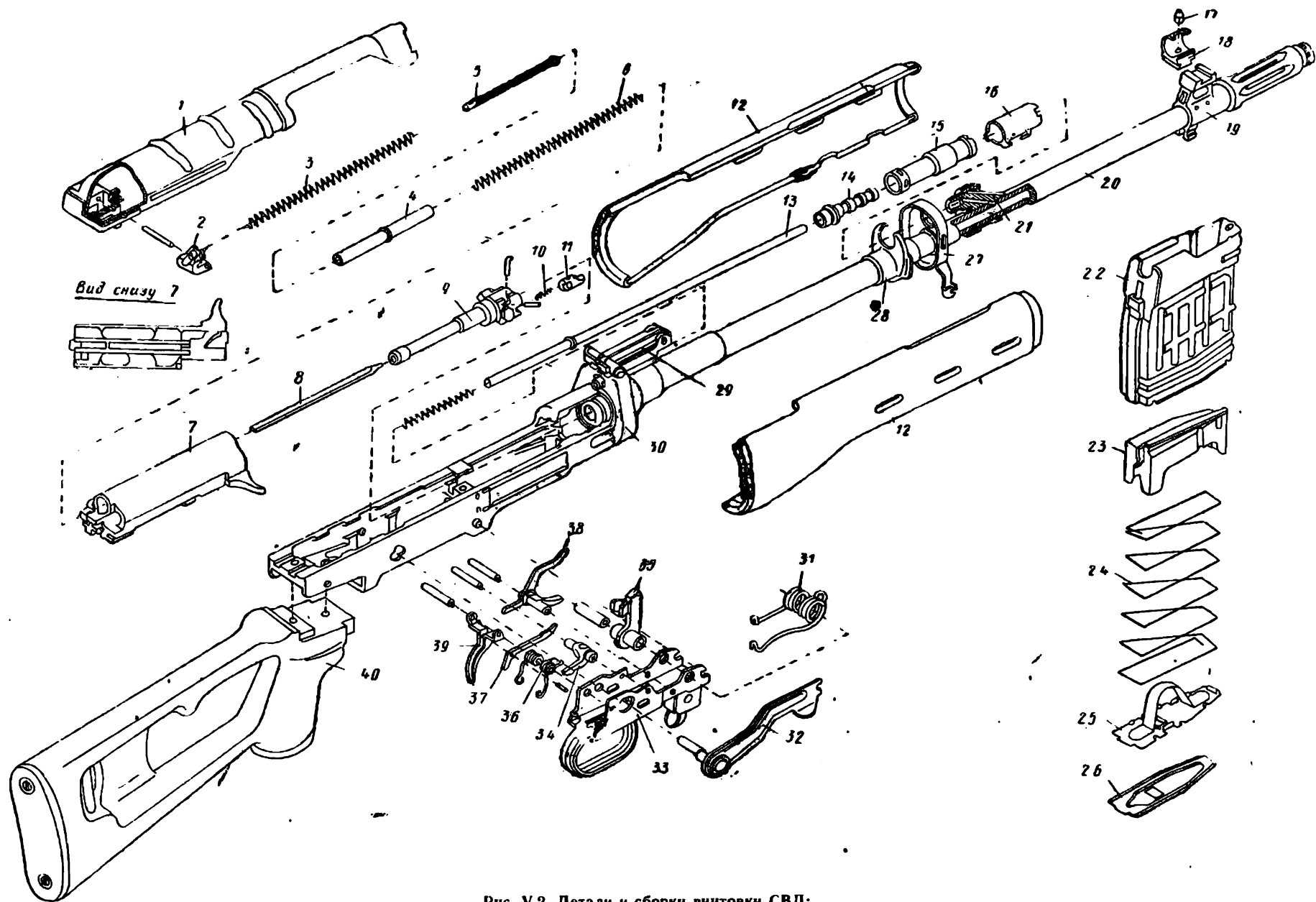
Рис. V.2. Детали и сборки винтовки СВД:
