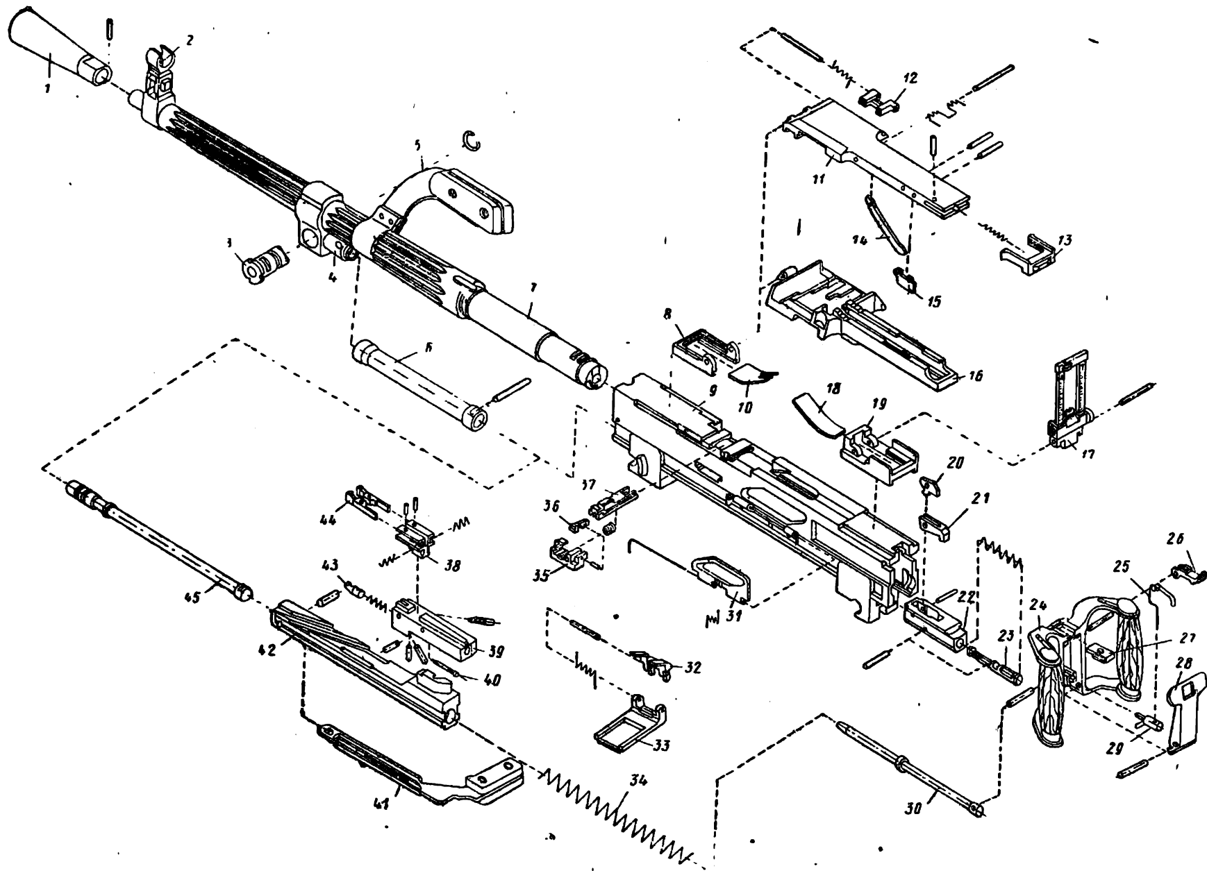
Рис. VI.4. Детали и сборки пулемета СГМ:
