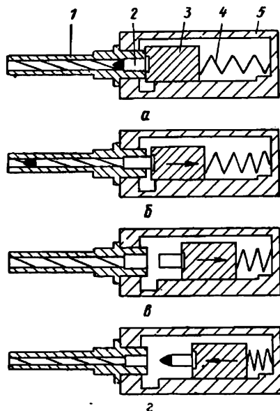
Рис. 1.19. Схема автоматического оружия, работающего на принципе отдачи свободного затвора (первый класс, 1-я группа, тип А):
