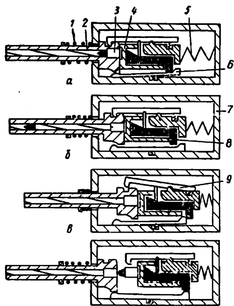
Рис. 1.22. Схема автоматического оружия, работающего на принципе отдачи ствола при длинном ходе: 1 — возвратная пружина ствола; 2 — ствол; 3 — гильза патрона; 4 — затвор; 5 — возвратная пружина затвора; 6 — автоматическое шептало; 7 — ствольная коробка; 8 — механизм отпирания; 9 — запирающий рычаг; а — положение в момент разбития капсюля; б — движение пули по каналу ствола; в — момент отпирания (в начале наката ствола); г — накат затвора
