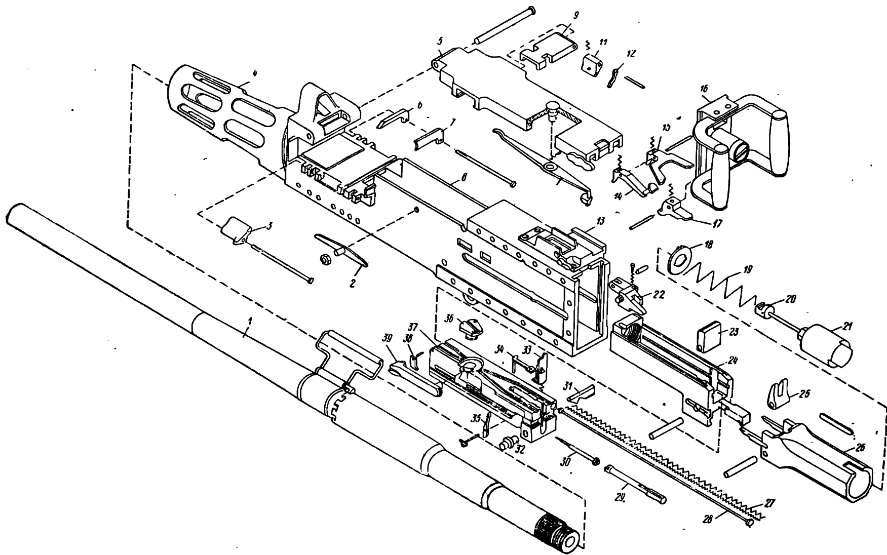
Рис. VII.6. Детали и сборки пулемета Браунинга (М2НВ):
