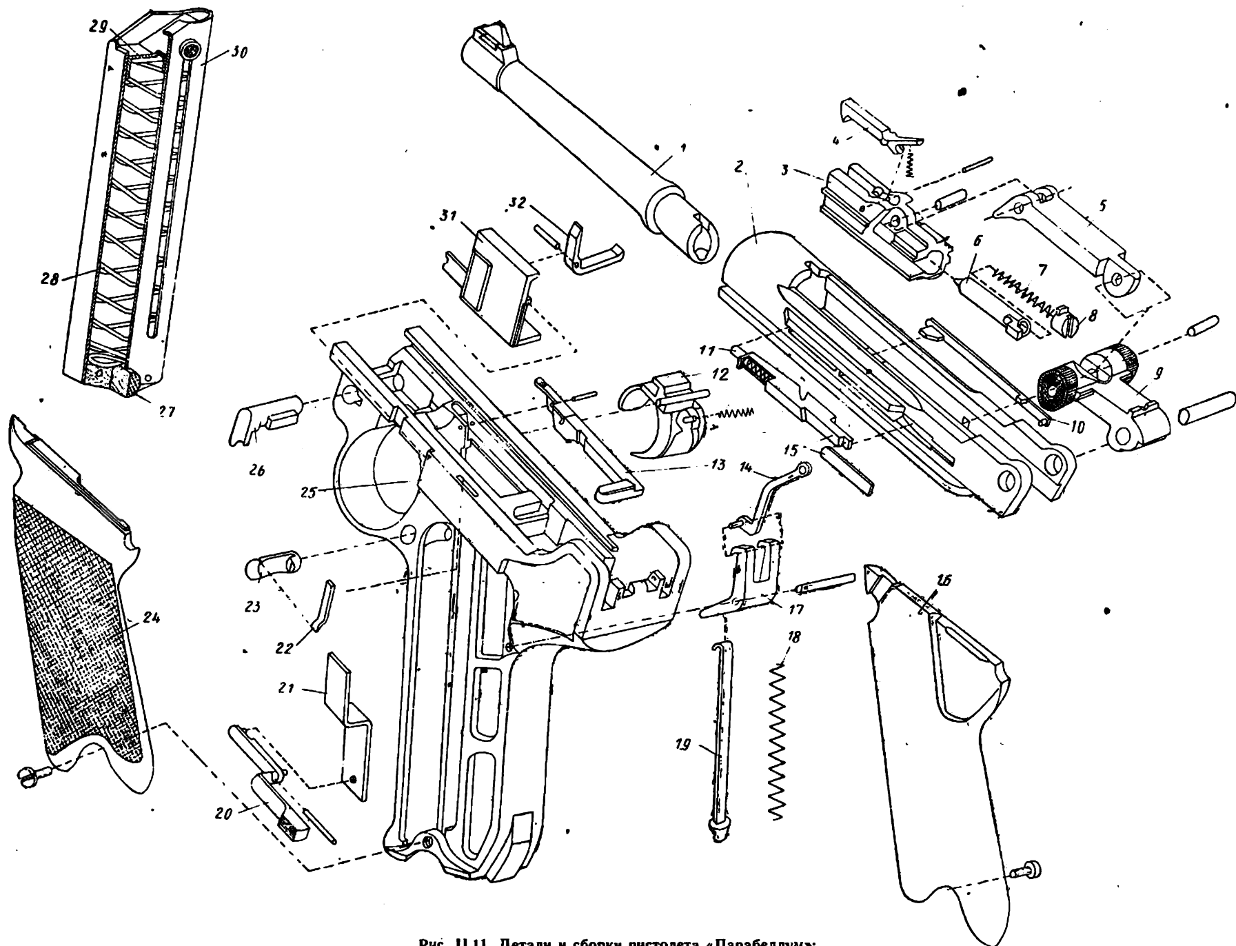
Рис. П.11. Детали и сборки пистолета «Парабеллум»:
