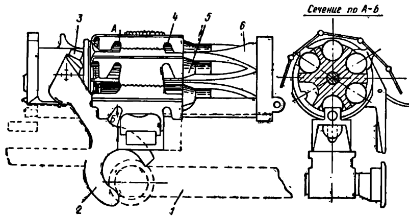
Рис. I.10. Конструктивная схема барабанного механизма подачи ленты: 1 — затворная рама; 2 — передаточный рычаг; 3 — храповое устройство; 4 — лента; 5 — патрон; 6 — барабан
