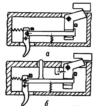
Рис. 1.5. Схемы спусковых механизмов:
