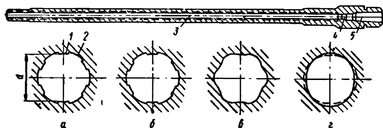
Рис. 1.1. Устройство ствола и его нарезной части: 1 - поле; 2 - нарез; 3 - нарезная часть; 4 - пульный вход; 5 - патронник; а, б, в, г - прямоугольный, трапециевидный, сегментный и овальный нарезы соответственно
