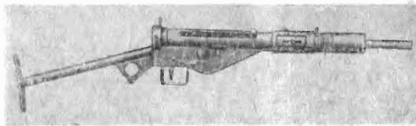
Рис. III.5. Pistolет-пулемет «Стен»
