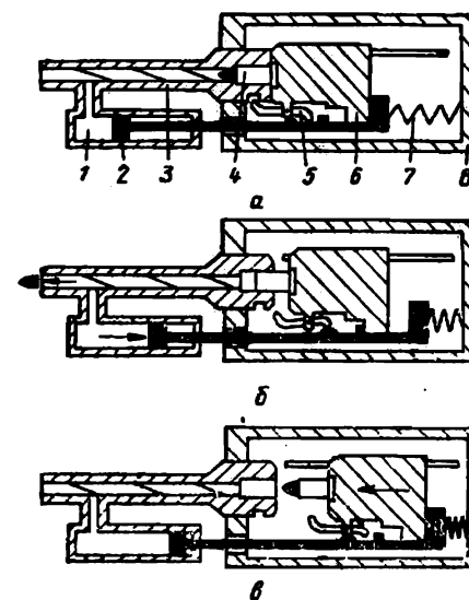
Рис. 1.24. Схема автоматического оружия, работающего на принципе отвода части пороховых газов через отверстие в стволе: 1 — газовая камера; 2 — поршень с затворной рамой; 3 — ствол; 4 — патрон; 5 — запирающий рычаг; 6 — затвор; 7 — возвратная пружина; 8 — ствольная коробка; а — положение в момент разбития капсюля; б — вылет пули из канала ствола; в — накат затвора
