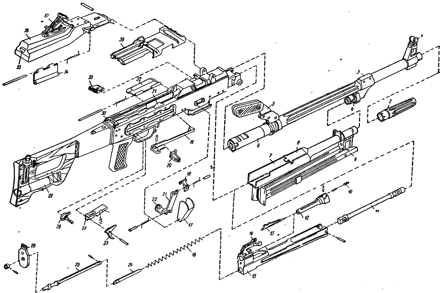
Рис. VI.16. Детали и сборки пулемета ПК:
