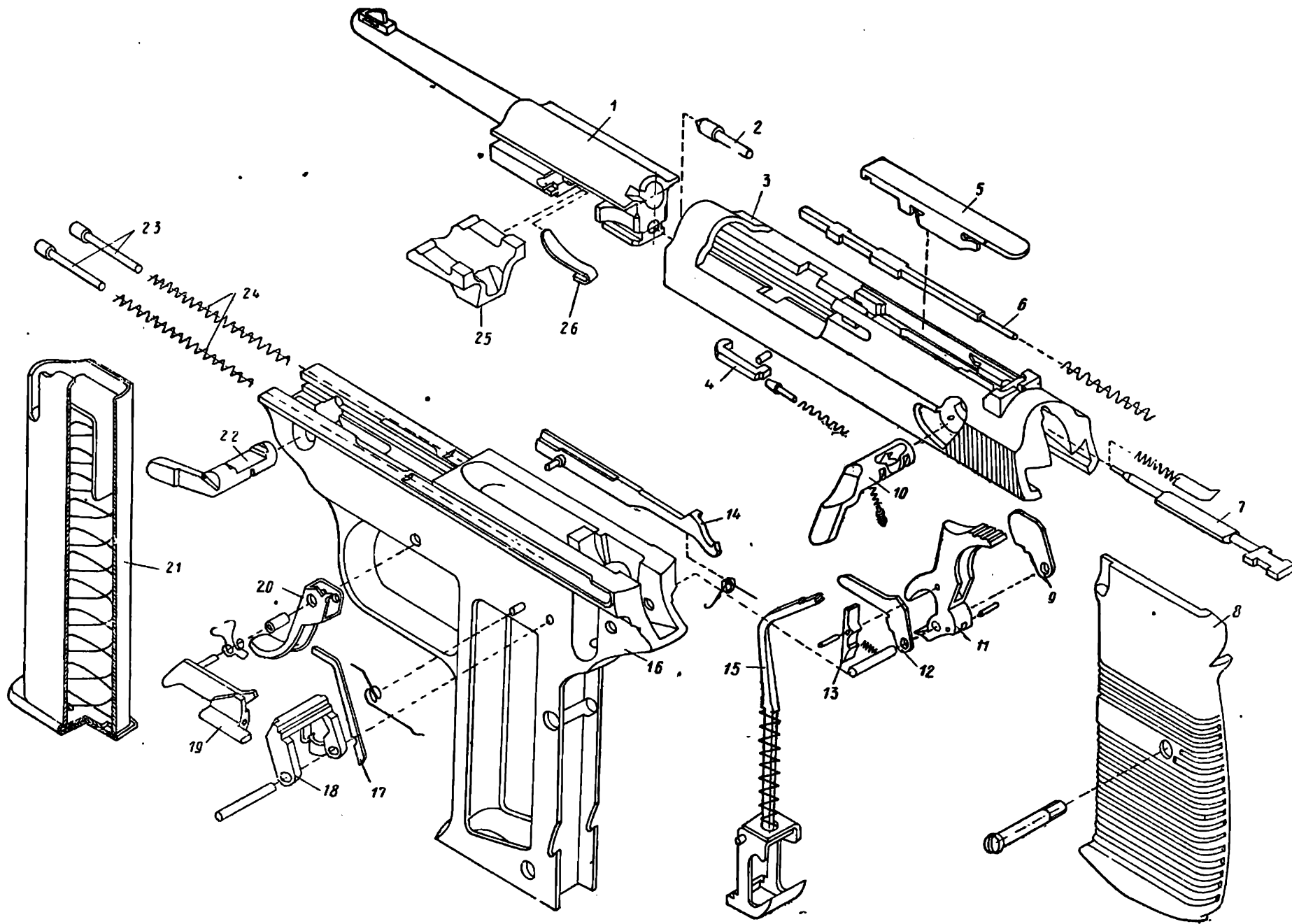
Рис. 11.9. Детали и сборки пистолета Вальтера:
