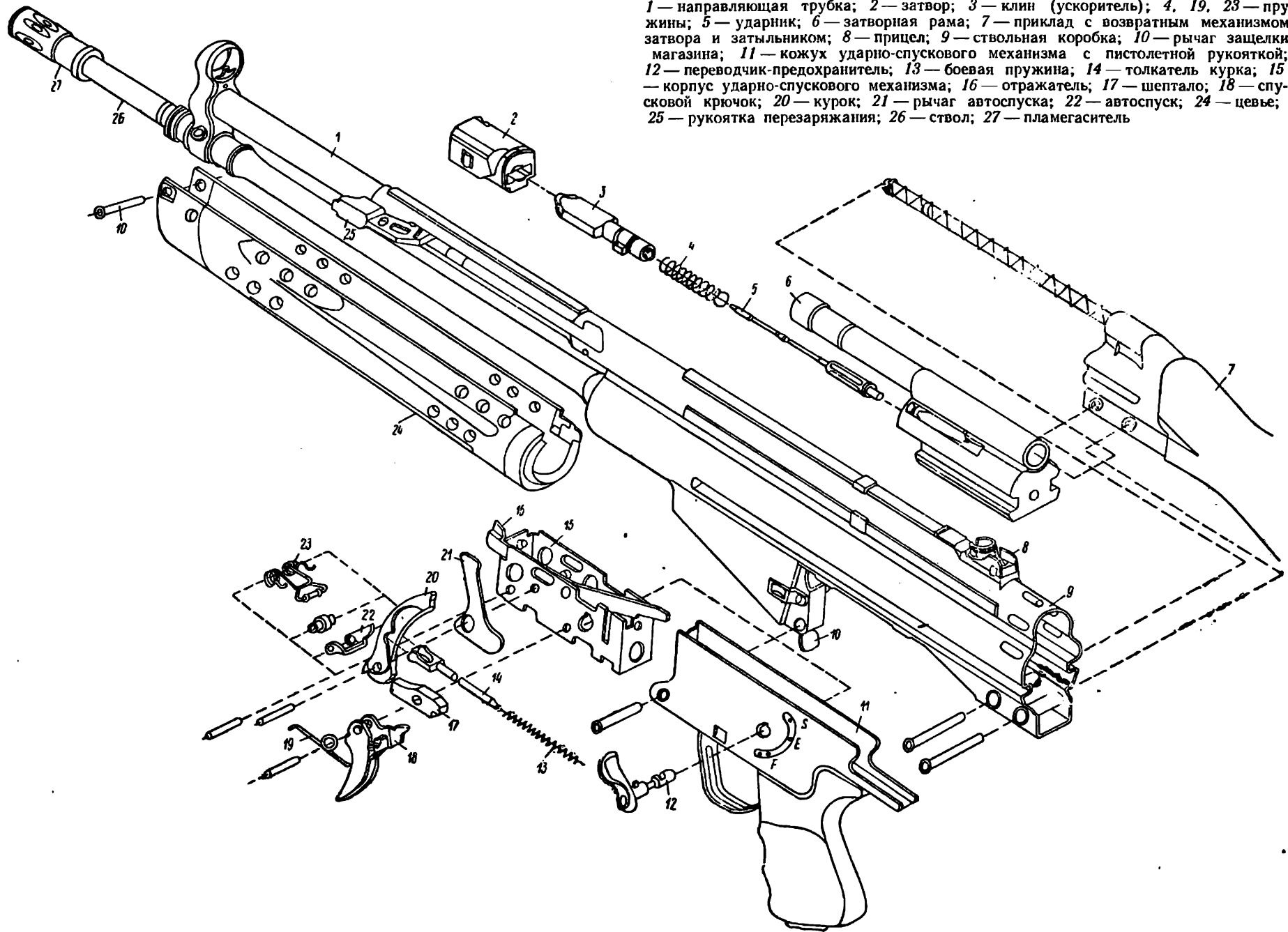
Рис. V.10. Детали и сборки винтовки G3
